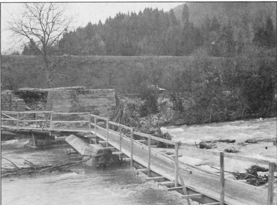
Slika 11. Zasilna lesena brv čez Savinjo ob 1. novembra porušenem savinskem mostu. Narasla reka jo je 26. novembra odnesla, kmalu za tem pa so začasno postavili trdnejši most iz beton- skih plošč; sedaj je na mestu starega že zgrajen nov železobetonski most.
