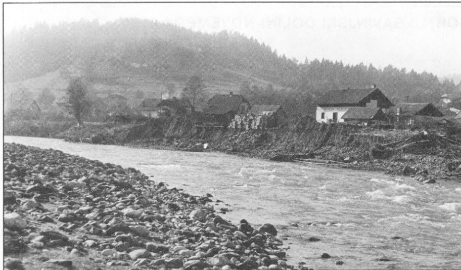
Slika 22. Porušeni del regulirane leve brežine Savinje v Mozirski kotlinici.
