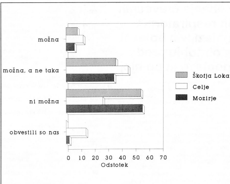
Slika 1. Pričakovanoost poplave.
