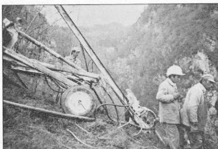
Slika 3. Sanacija kameninskega podora se je pričela marca 1989. Vsa oprema je bila s helikopterji JLA in RSNZ iz Ljubljane prepeljana na greben nad odlomom. Dokumentacija MMI.
