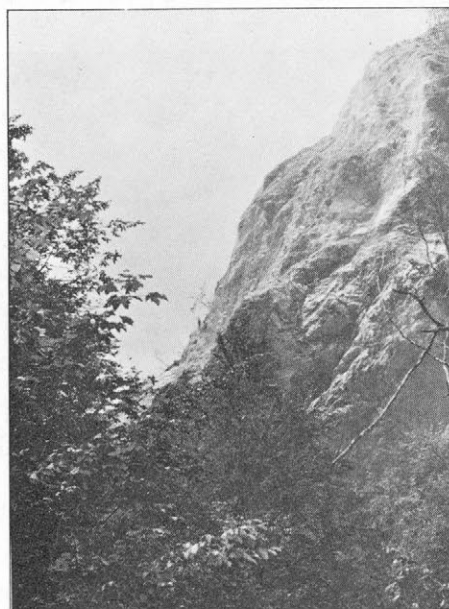
Slika 5. Prikazano je miniranje zgornjega odlomnega roba. Dokumentacija GZL.
