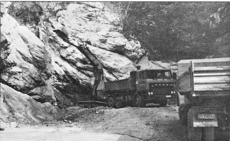
Slika 13. Konec oktobra in v začetku novembra 1989 je bilo z območja podslapja v soteski Pasice na dolžini približno 200 metrov s kamioni odpeljano približno 15 000 m 3 materiala. Dokumentacija MMI.
