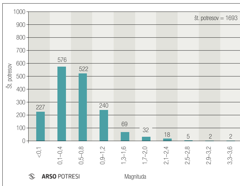
Slika 3: Porazdelitev magnitude ( M_{LV} ) potresov v Sloveniji leta 2018
