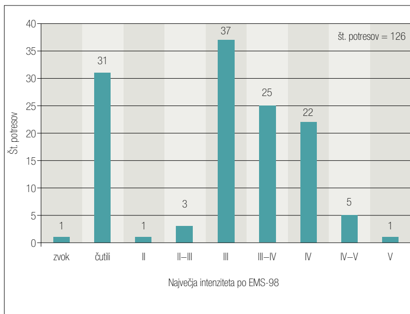
Slika 9: Porazdelitev največje intenzitete po EMS-98 potresov v Sloveniji leta 2018
